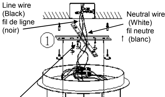
Ground wire (Copper or Green) fil de mise à la terre (cuivre ou vert)
